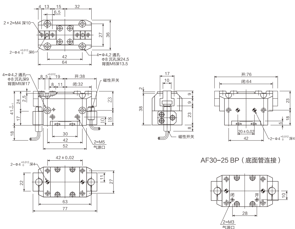
外形尺寸图
